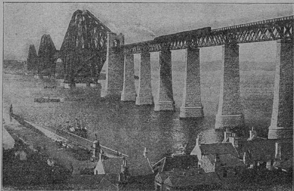
Желѣзно-дорожный мостъ черезъ заливъ Фортъ.
