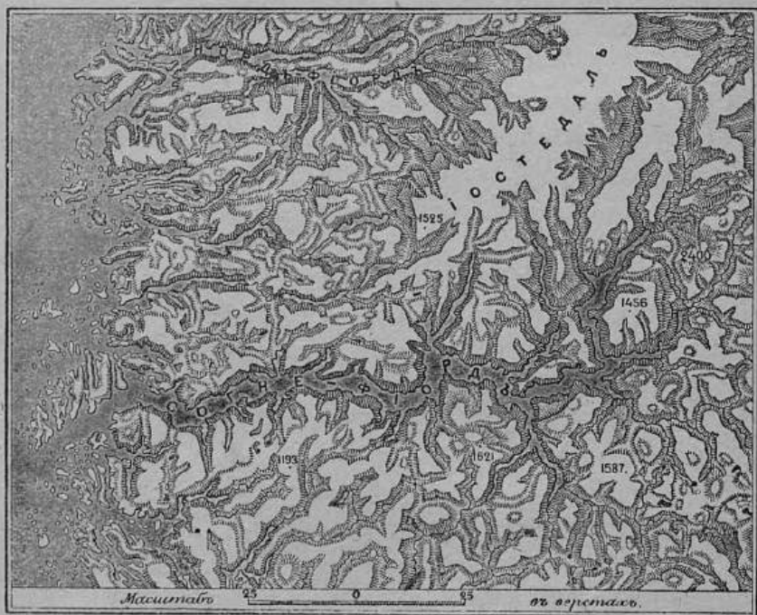
Карта Согне-фіорда.
