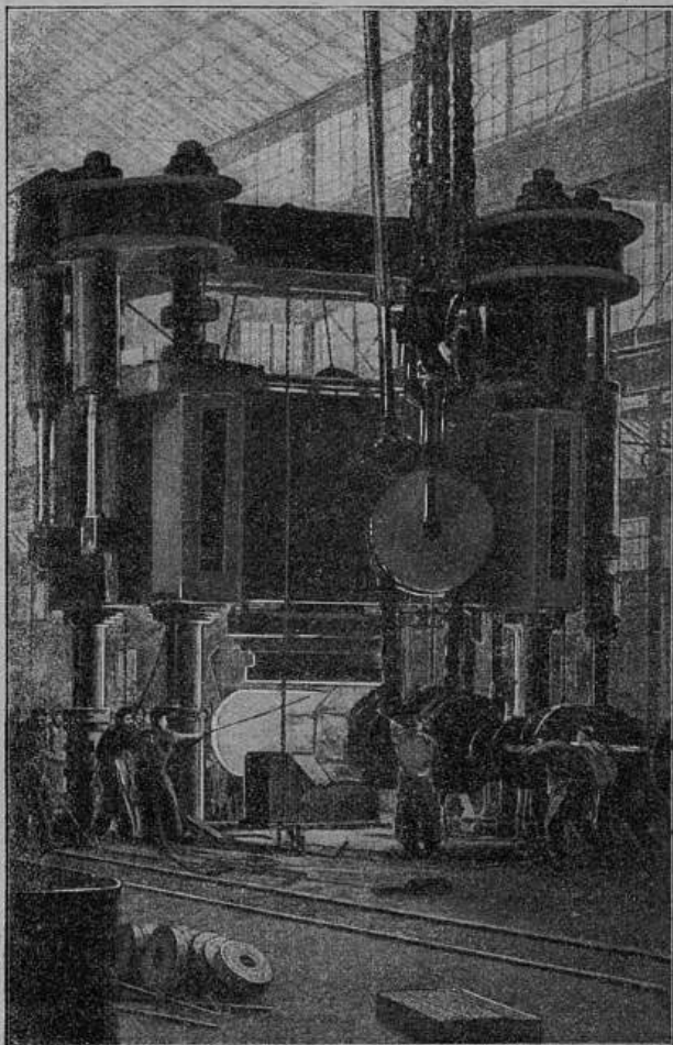
Выдѣлка стальной оси для корабельнаго винта, на Крупповскомъ заводѣ. Раскаленная ось находится подъ прессомъ, который давитъ съ силою 300.000 пудовъ.
