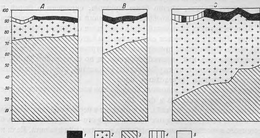
Фиг. 10. Основные компоненты современных глубоководных осадков.
