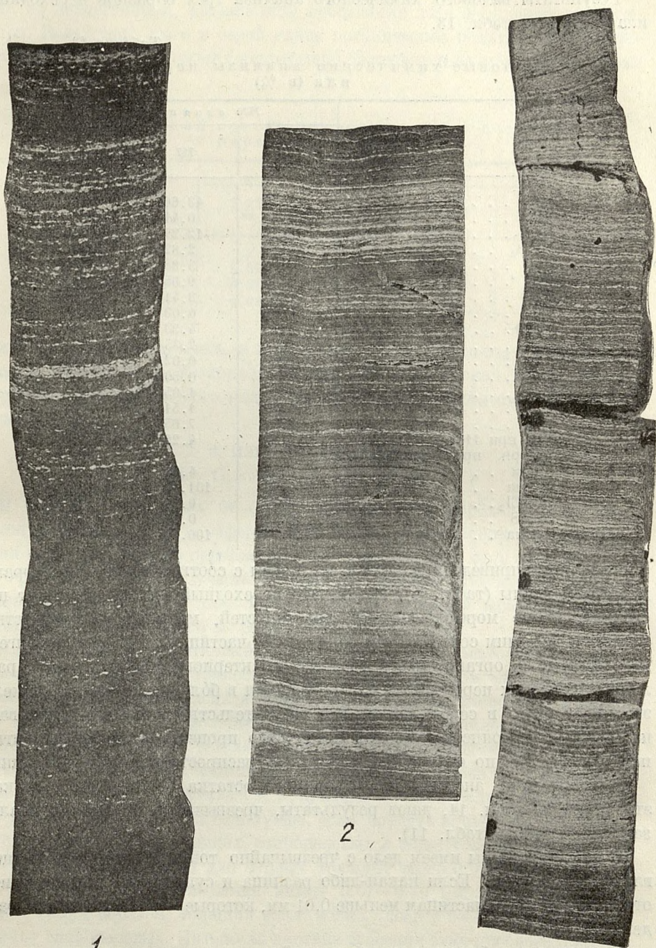
Фиг. 11. Основные разности переходного глубоководного ила и известковый ил.
